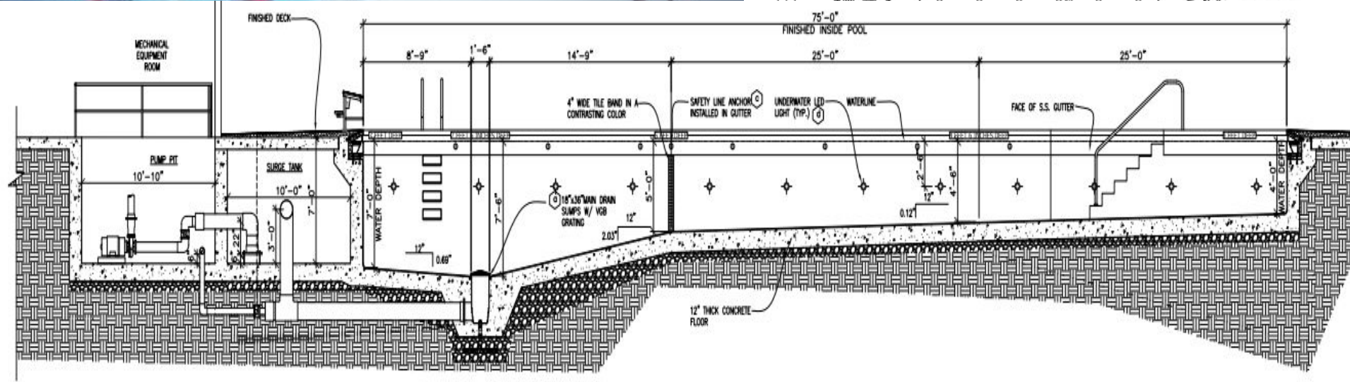
1 POOL LONGITUDINAL SECTION
